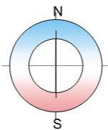
径向充磁
