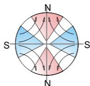
外圆多极充磁
