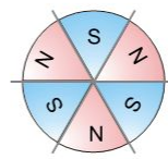
轴向多极充磁
